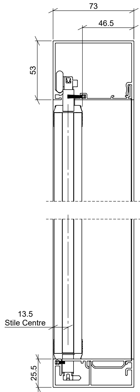
SECTION A-A
